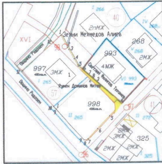
ПЛАН ЗА РЕГУЛАЦИЯ М 1:500
